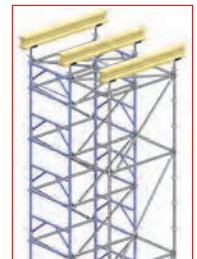
Torre con extensión Allround
