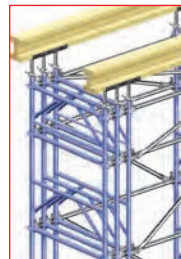
Marcos agrupados para aumentar la capacidad de carga
