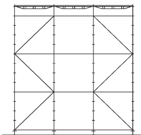
Sección A-A
