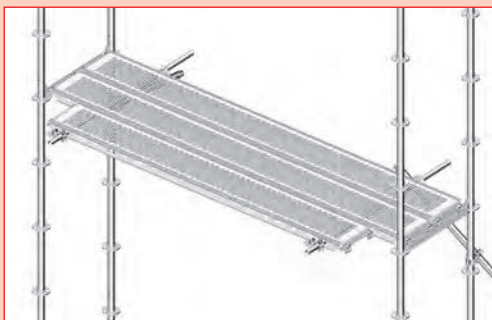
▶ Plataforma T9 en acero, de 0,19 m. de ancho
