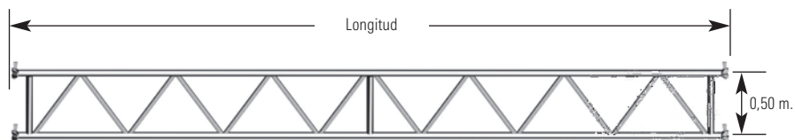
▶ Viga de celosía
