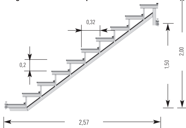
▶ Viga escalera 200 de 10 peldaños
