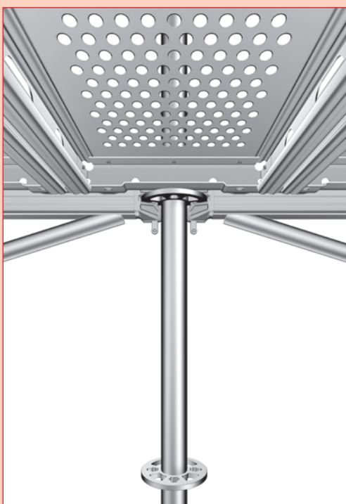
▶ Plataforma Robust, de 0,61 m. de ancho "U"
