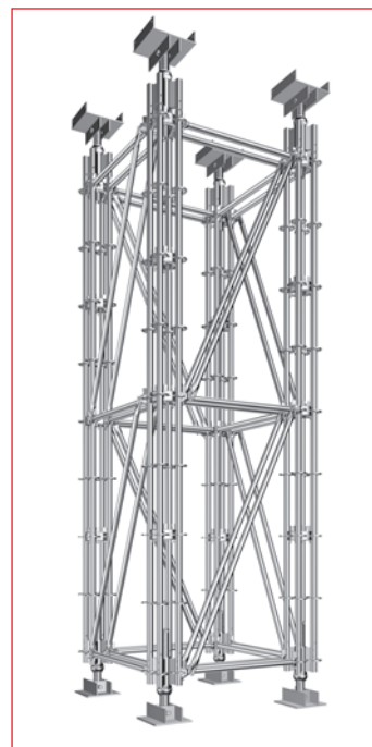
▶ Collarín cuádruple de alta resistencia
