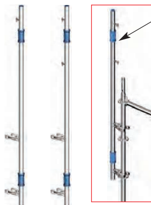
▶ Postes de montaje T5
