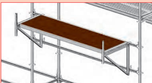
▶ Ménsula en "U", de 1,09 m.
