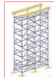
Torre con múltiples planos de marcos
