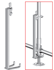
► Cabezal de cimbra 45/60, macizo de 16 cm.
