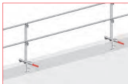
Ejemplo de aplicación de la mordaza para forjado en petos
