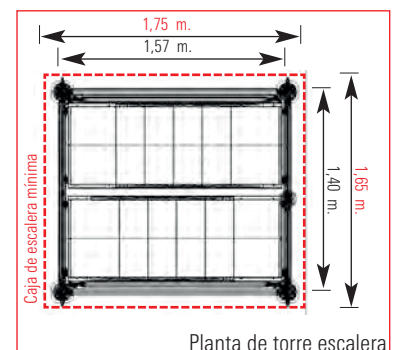
Planta de torre escalera
