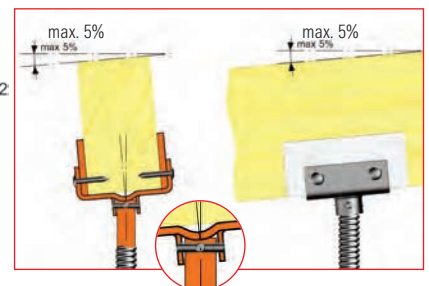
► Cabezal de cimbra 45/60, de inclinación variable macizo de 16 cm.
