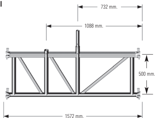
▶ Viga peatonal
